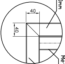
DETALHE A
