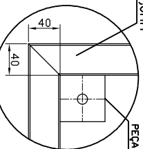
DETALHE C
