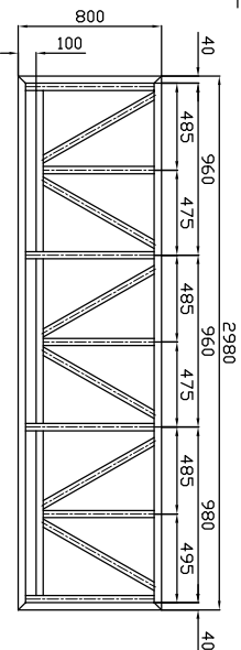
VISTA INFERIOR
